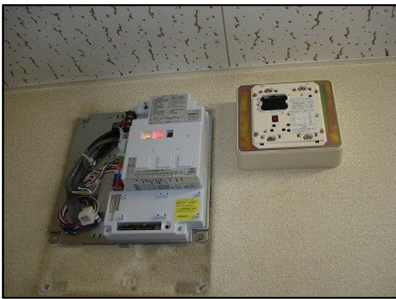
制御盤とテンキー制御器(親) 結線取替中。
