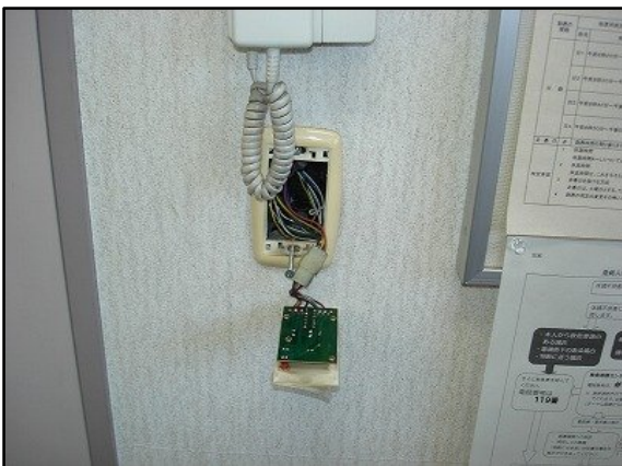
遠隔解錠出来る 操作表示器 交換中 管理室、インタホンと連動
