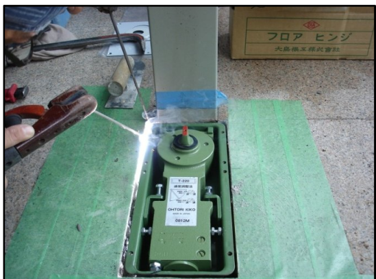
セメント箱を溶接
